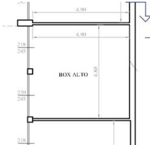
PIANTA BOX AUTO DI CUI AL MAPPALE 752 SUB. 507
