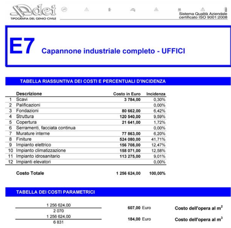
Fig. 3 – Valori parametrici costo di costruzione uffici (da “Prezzi Tipologie Edilizie” DEI Tipografia del Genio Civile, ed. 2014)
