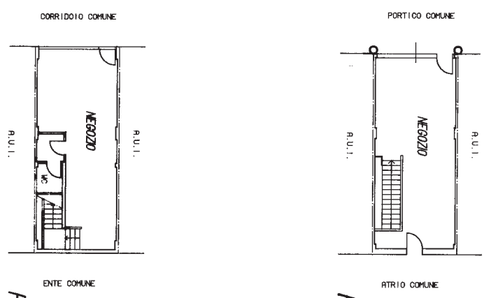
PIANTINA P.T. (H=370) PIANTINA P.1.S. (H=290)
