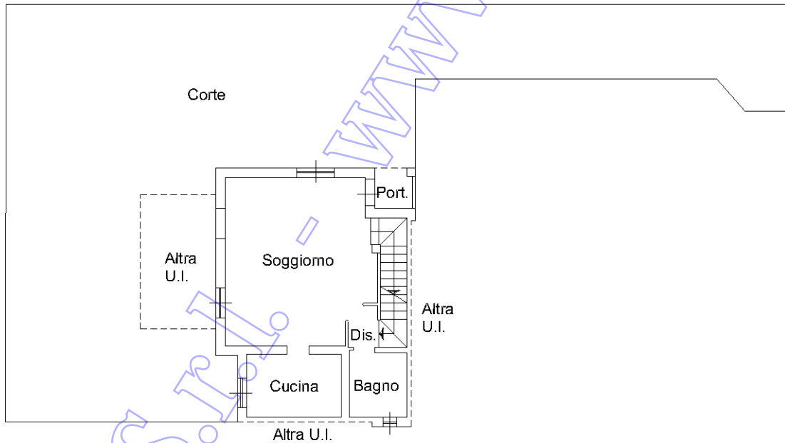
PIANTA PIANO TERRA H=2.55 m.
