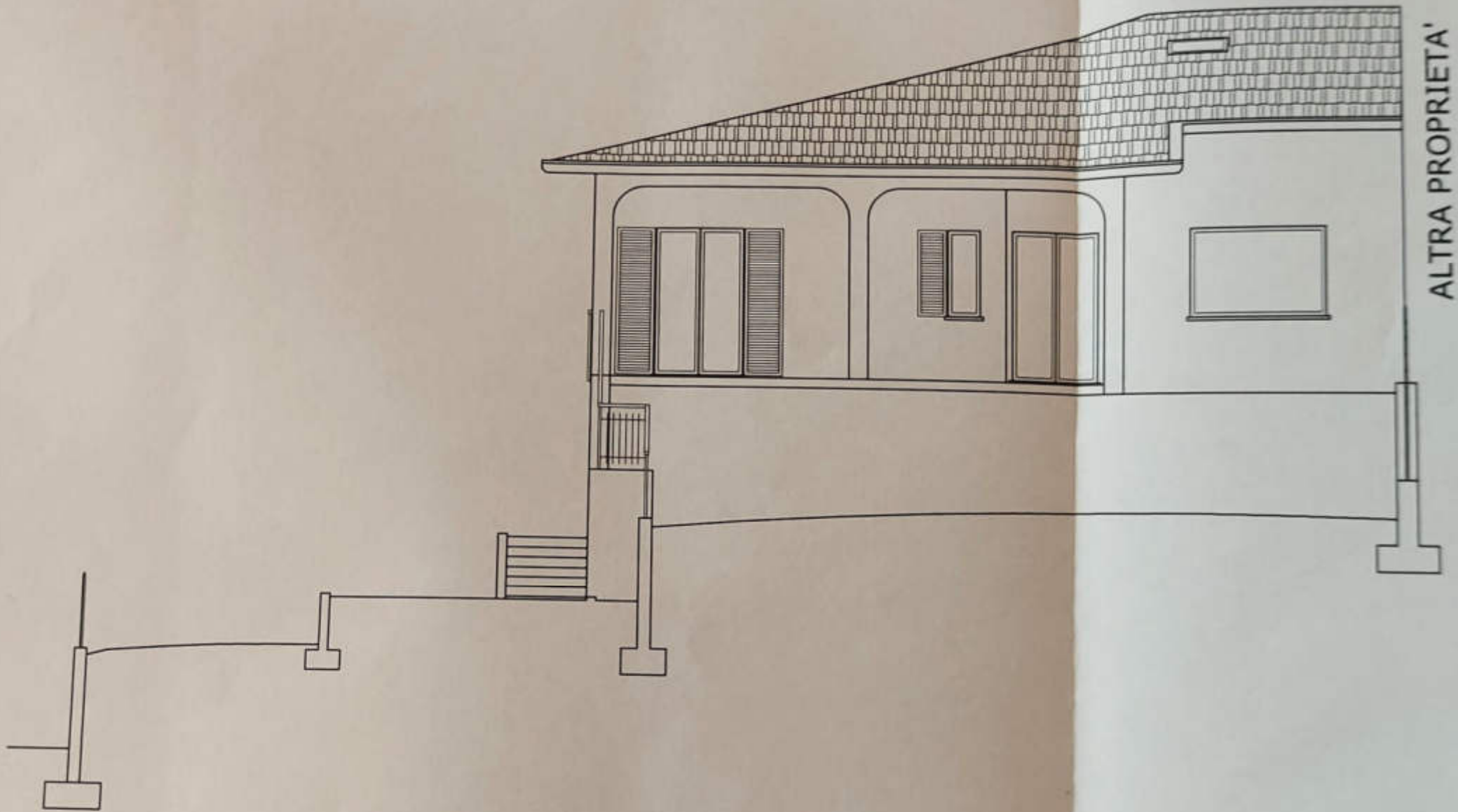
PROSPETTO EST (D-D)
