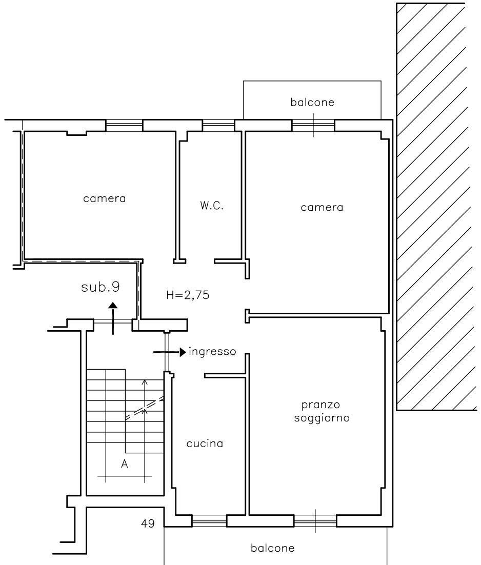
PIANO TERZO sc. 1:100
