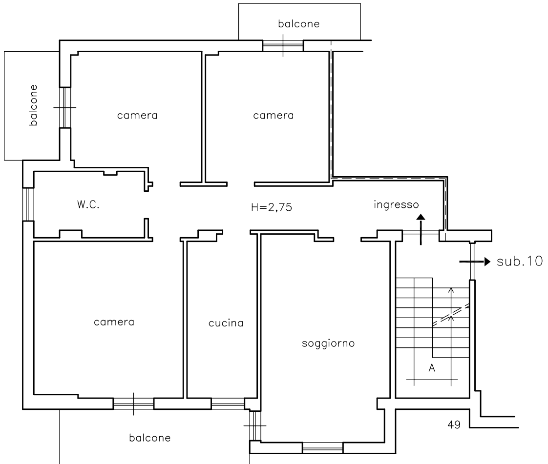
PIANO TERZO sc. 1:100
