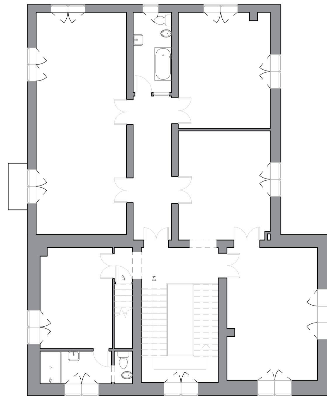
PIANO FONDI h 3,65
