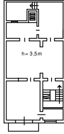
piano primo
