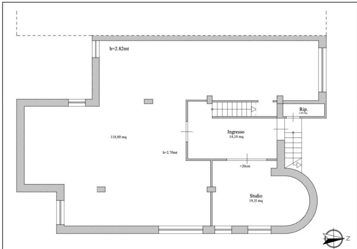
Figura 6 – Grafico dello stato dei luoghi – piano seminterrato
