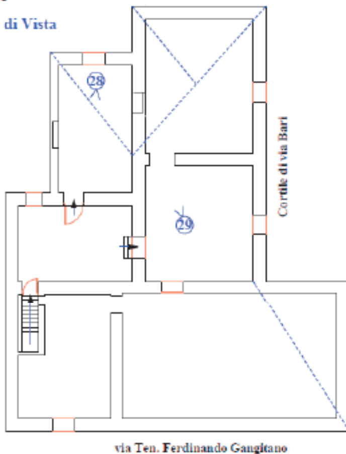
Pianta Sottotetto
