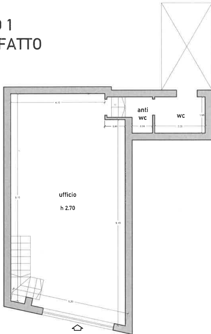
PIANO TERRA PIANTA STATO ATTUALE Scala 1:100
