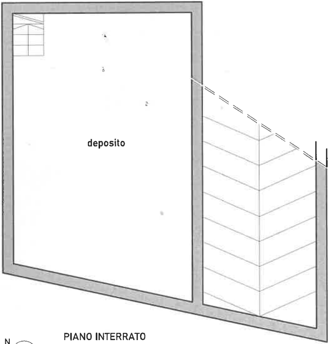
PIANO INTERRATO PIANTA STATO AUTORIZZATO Scala 1:100
