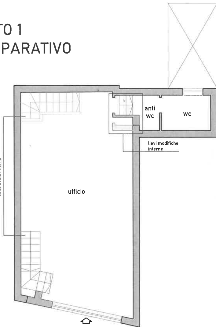
PIANO TERRA PIANTA STATO COMPARATIVO Scala 1:100
