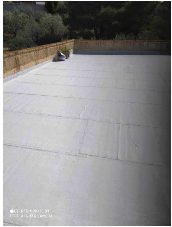
COPERTURAPIANA
