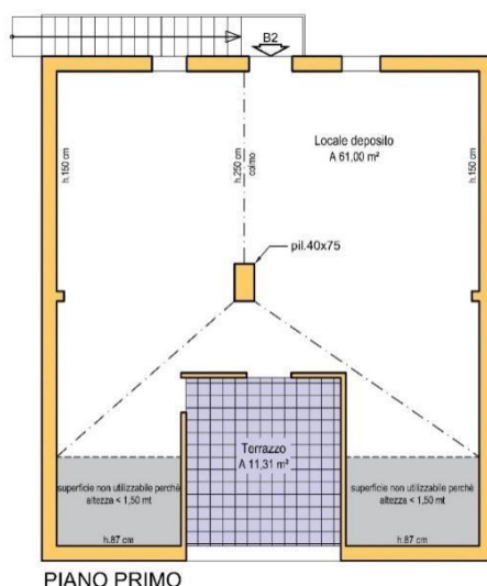
Pianta del Primo Piano (deposito sottotetto)
