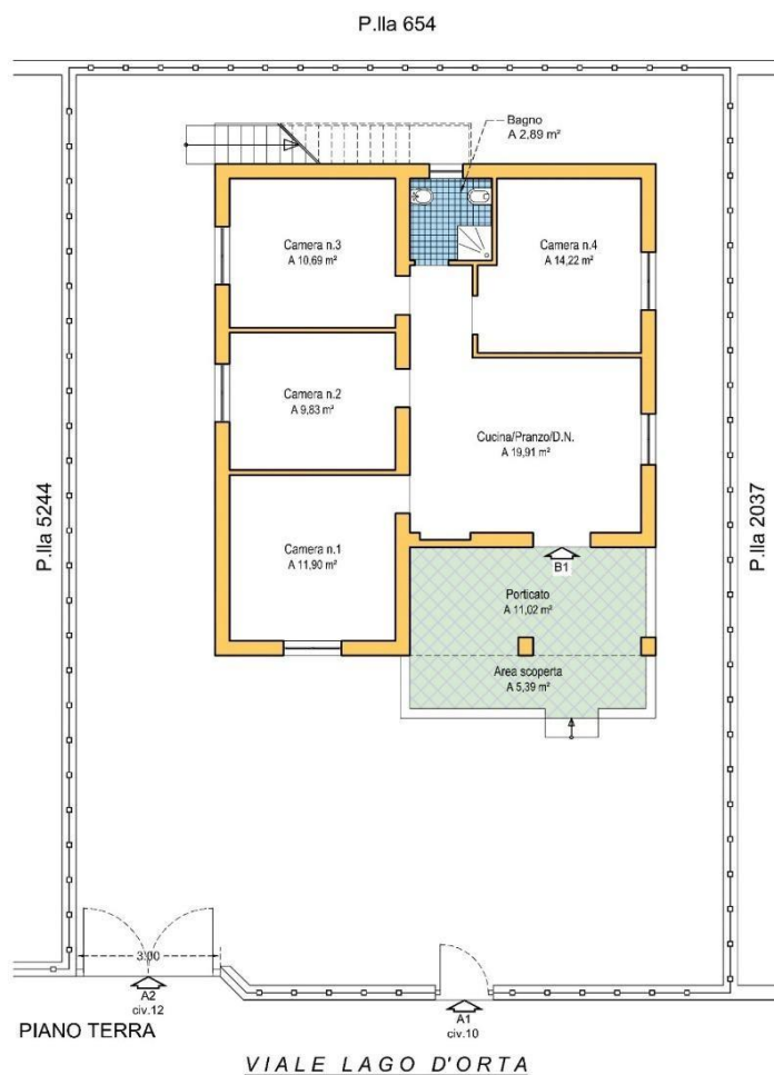
Pianta del Piano Terra alla data del sopralluogo
