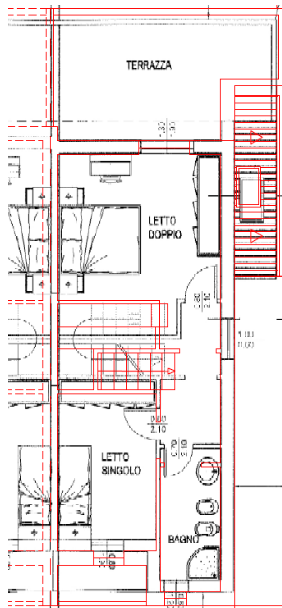
Figura 71 - Sovrapposizione progetto-rilievo. Piano 1, fuori scala
