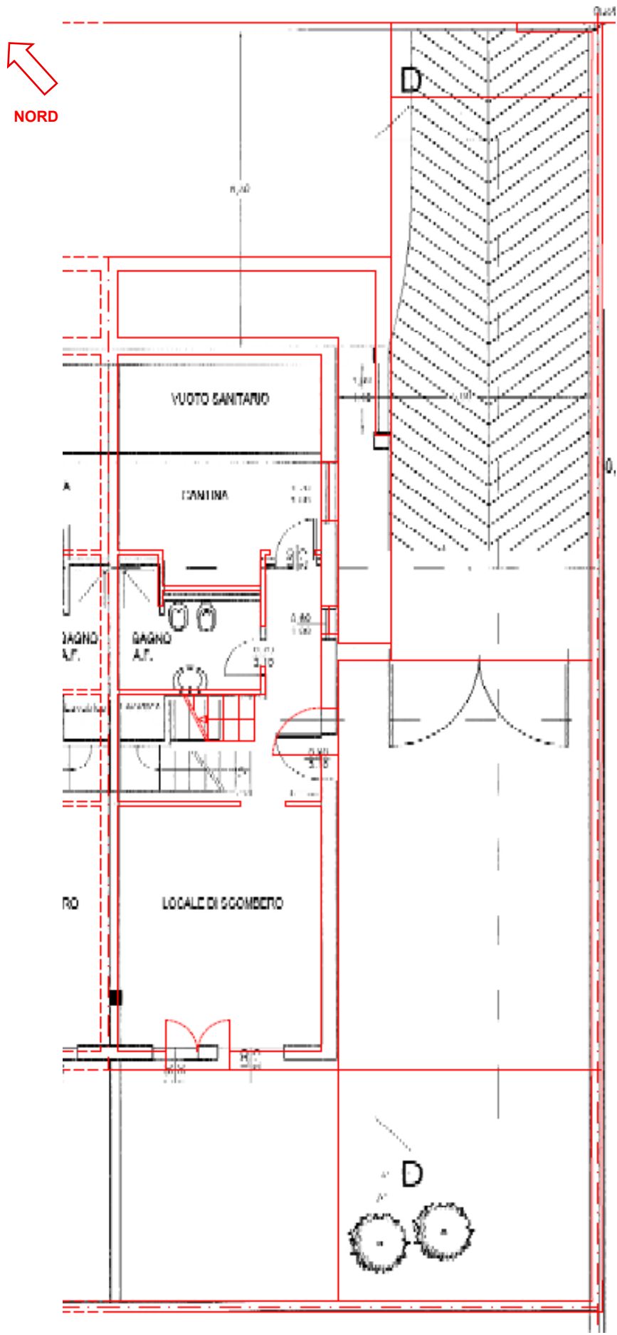
Figura 69 - Sovrapposizione progetto-rilievo. Piano S1, fuori scala
