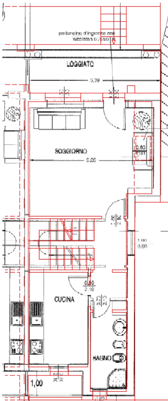
Figura 70 - Sovrapposizione progetto-rilievo. Piano T, fuori scala
