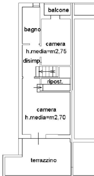
Figura 65 – Stralcio planimetria catastale in atti (fuori scala). Piano primo
