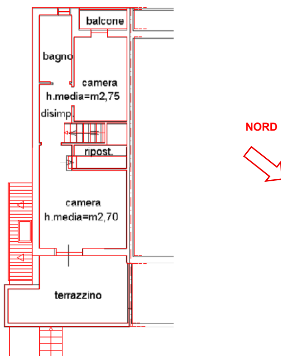
Figura 67 – Sovrapposizione rilievo con planimetria catastale in atti (fuori scala). Piano terra
