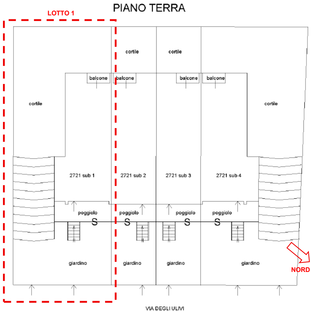
Figura 2- Stralcio dell'elaborato planimetrico (Piano T, fuori scala)
