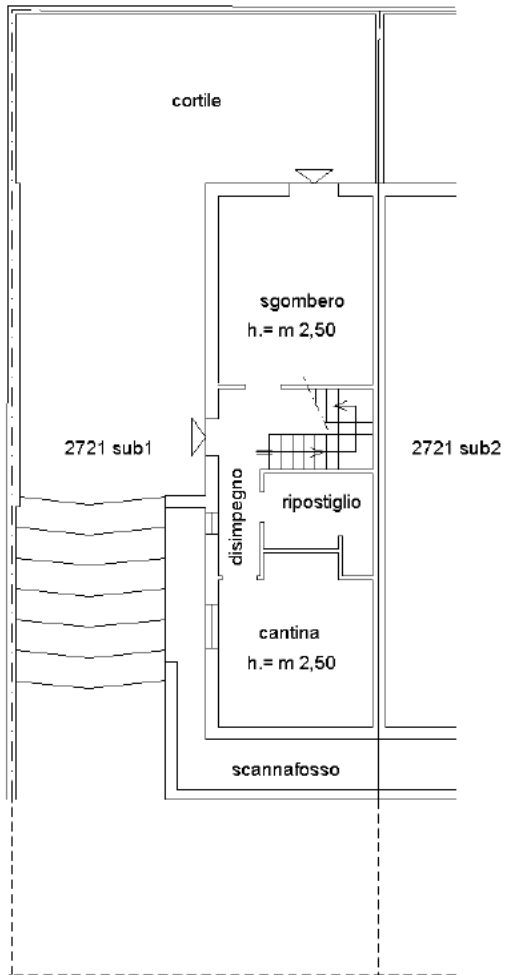
Figura 63 – Stralcio planimetria catastale in atti (fuori scala). Piano seminterrato
