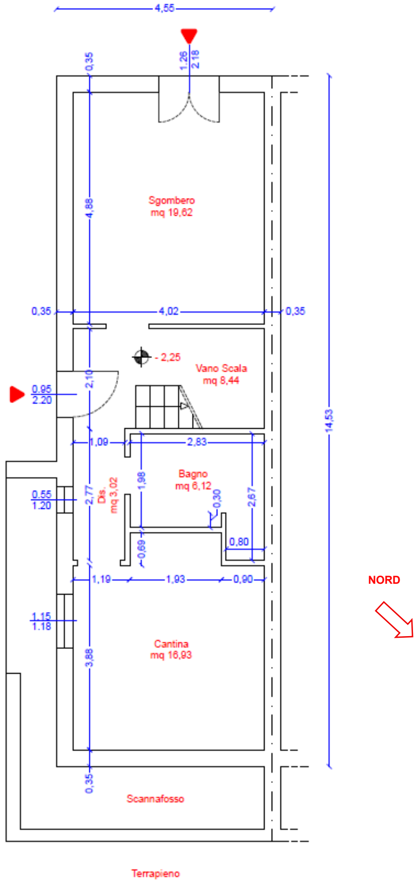
Figura 15 - Rilievo sub. 1 piano seminterrato, fuori scala. H mt 2,50
