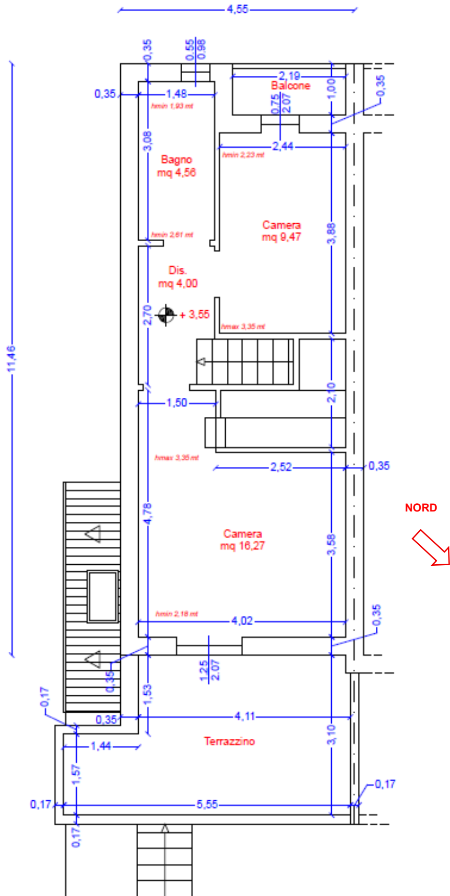
Figura 17 - Rilievo sub. 1 piano primo, fuori scala. H varie
