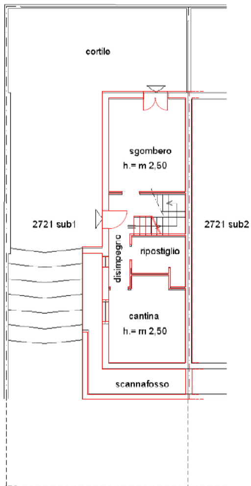
Figura 66 – Sovrapposizione rilievo con planimetria catastale in atti (fuori scala). Piano seminterrato
