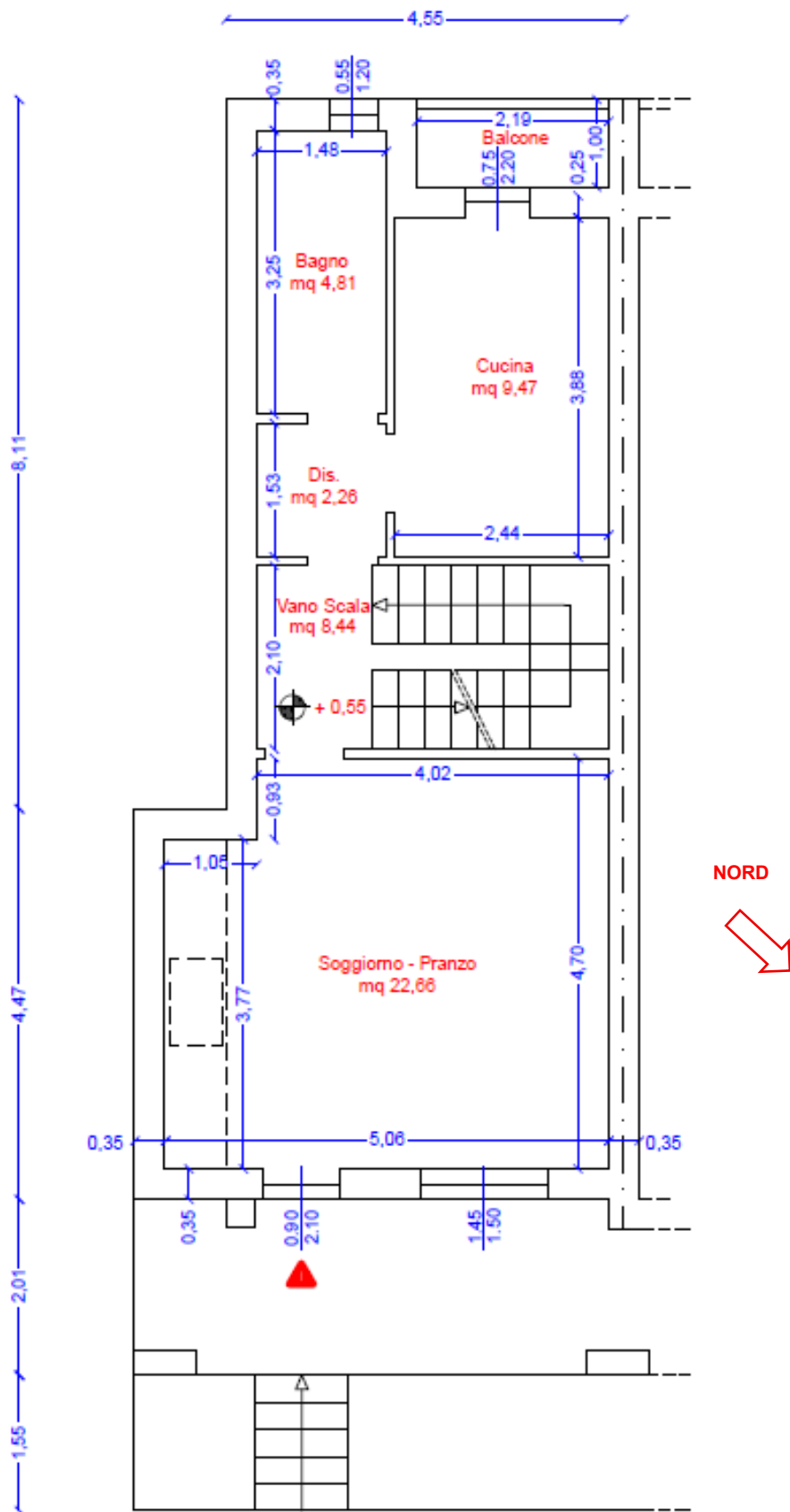
Figura 16 - Rilievo sub. 1 piano terra, fuori scala. H mt 2,70
