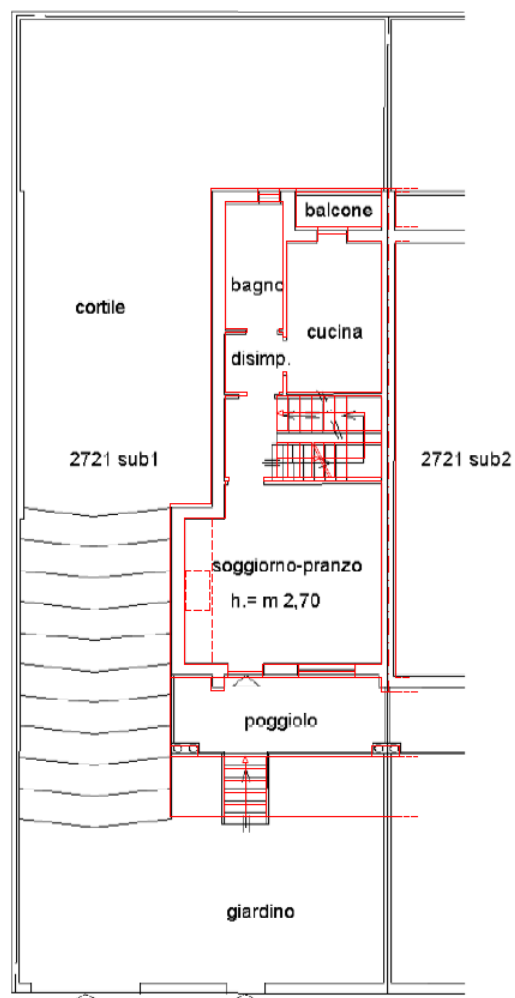
Figura 67 – Sovrapposizione rilievo con planimetria catastale in atti (fuori scala). Piano terra
