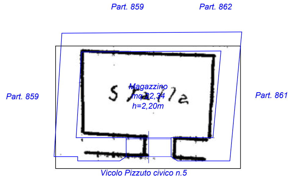
PIANTA STATO DI FATTO PIANO TERRA scala 1:100
