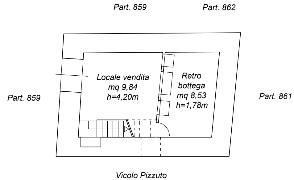
PIANTA STATO DI FATTO PIANO PRIMO scala 1:100
