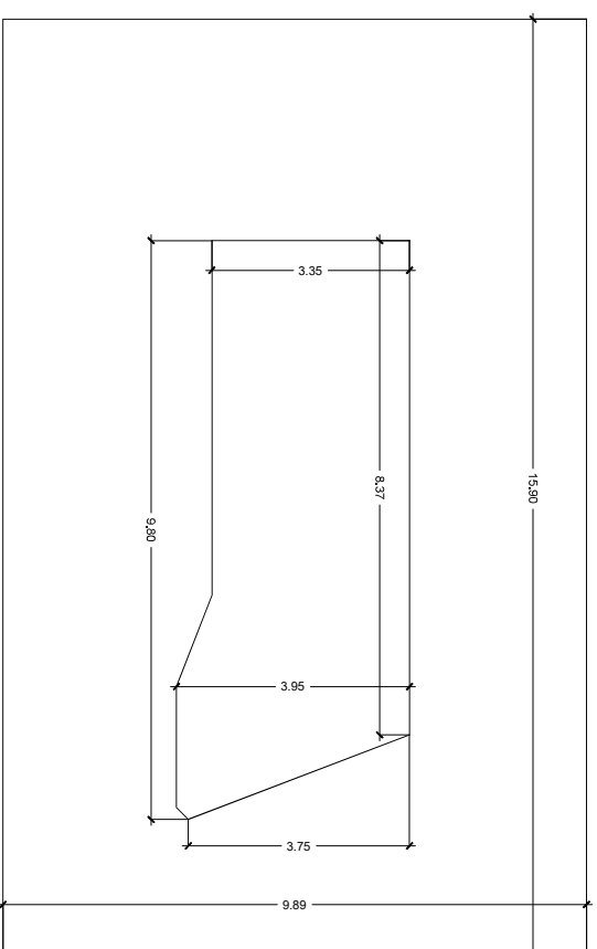
PIANTA PISCINA
