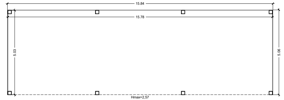
PIANTA PIANO TERRA
