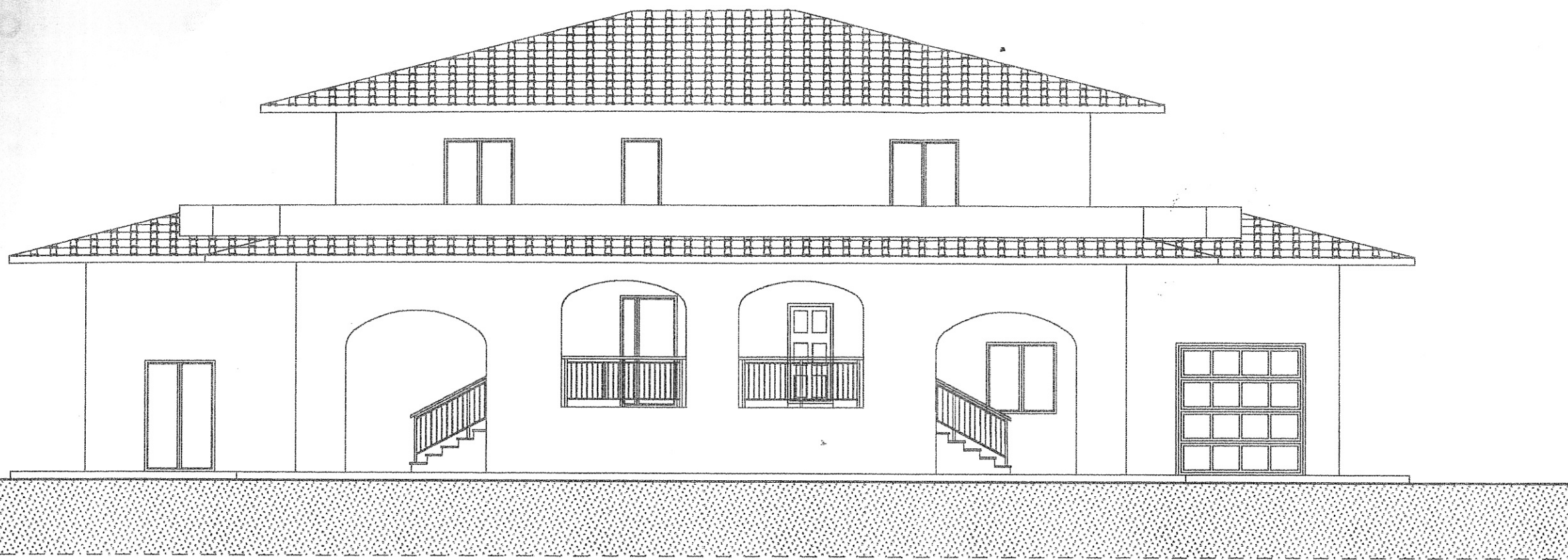
prospetto A/1
