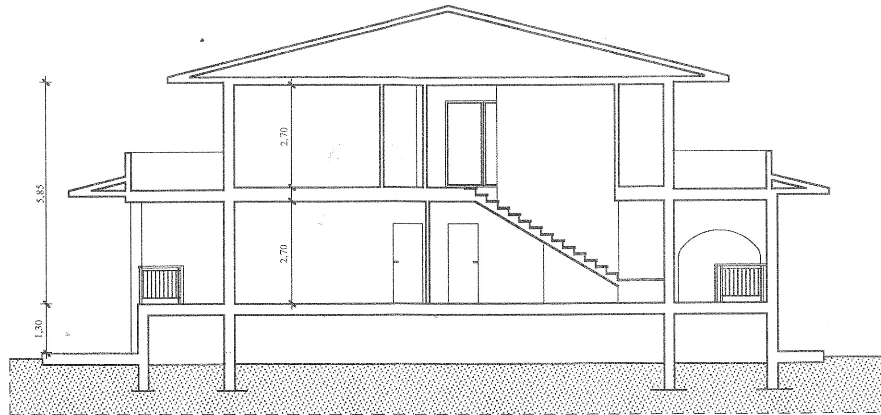
sezione S/2
