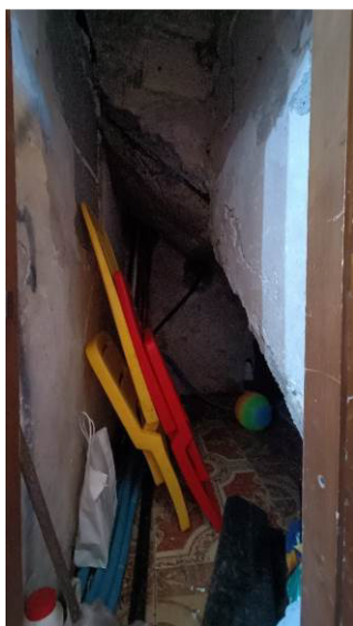
Umidità di risalita disimpegno sottoscala Ammaloramento soletta scala
