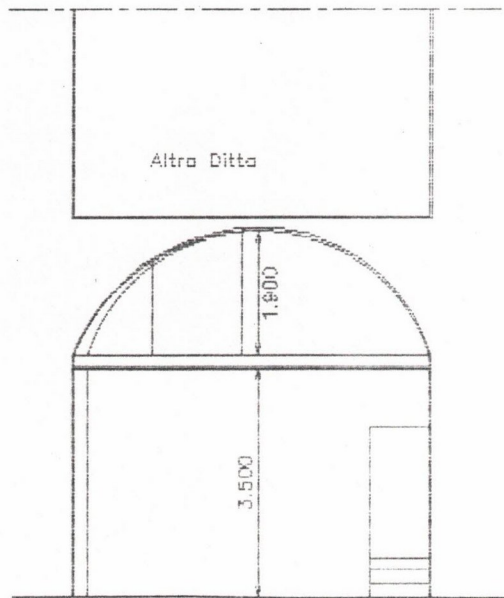
Sezione A-A
