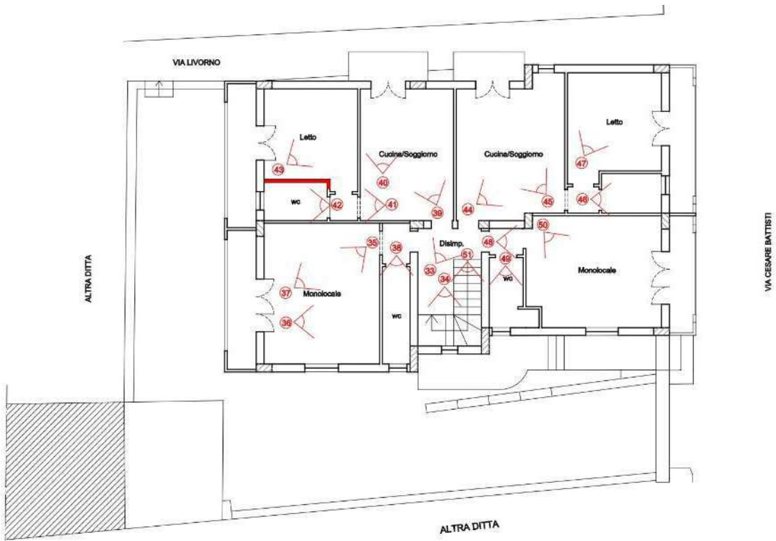
Pianta con ottici piano secondo
