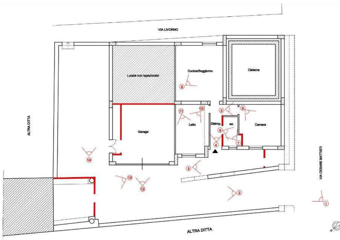
Pianta con ottici piano terra
