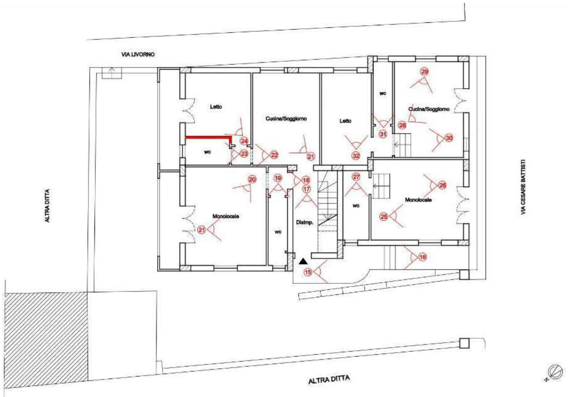
Pianta con ottici piano primo
