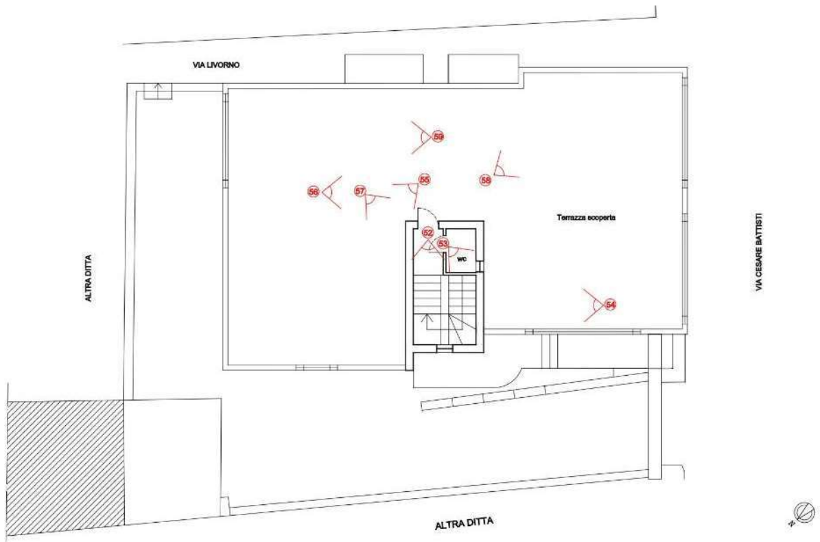
Pianta con ottici piano copertura
