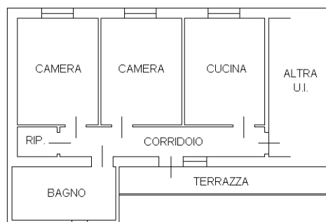
PIANTA PIANO PRIMO H=273
