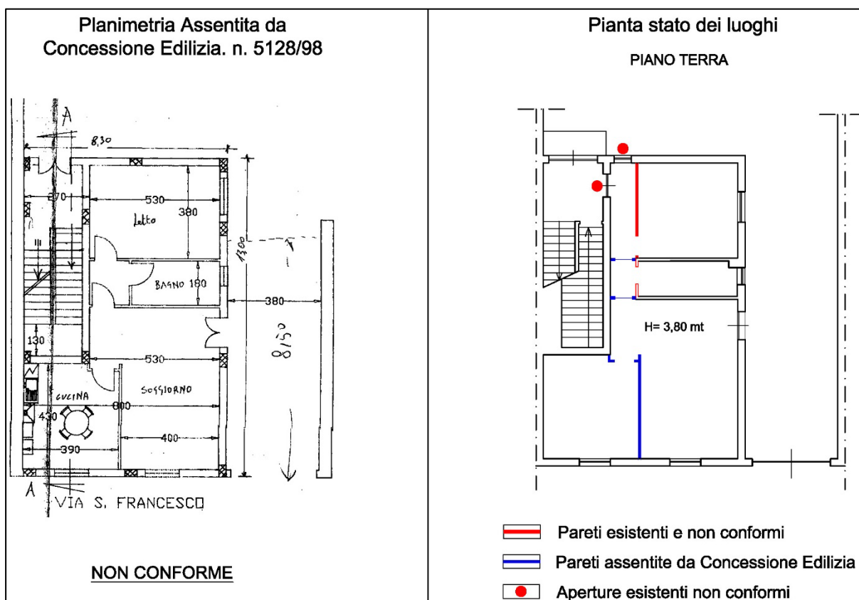
Fig. 6 - Planimetria delle Difformità Urbanistiche
