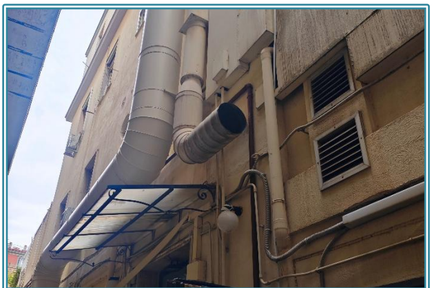
Figura 13 Particolare dell'impianto di areazione sulla facciata del fabbricato
