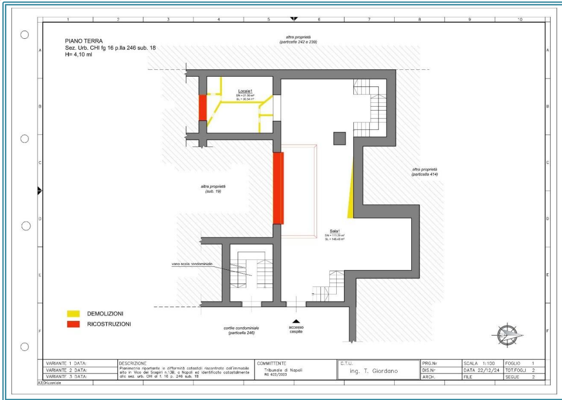
Figura 47 Schema difformità catastali – Piano Terra
