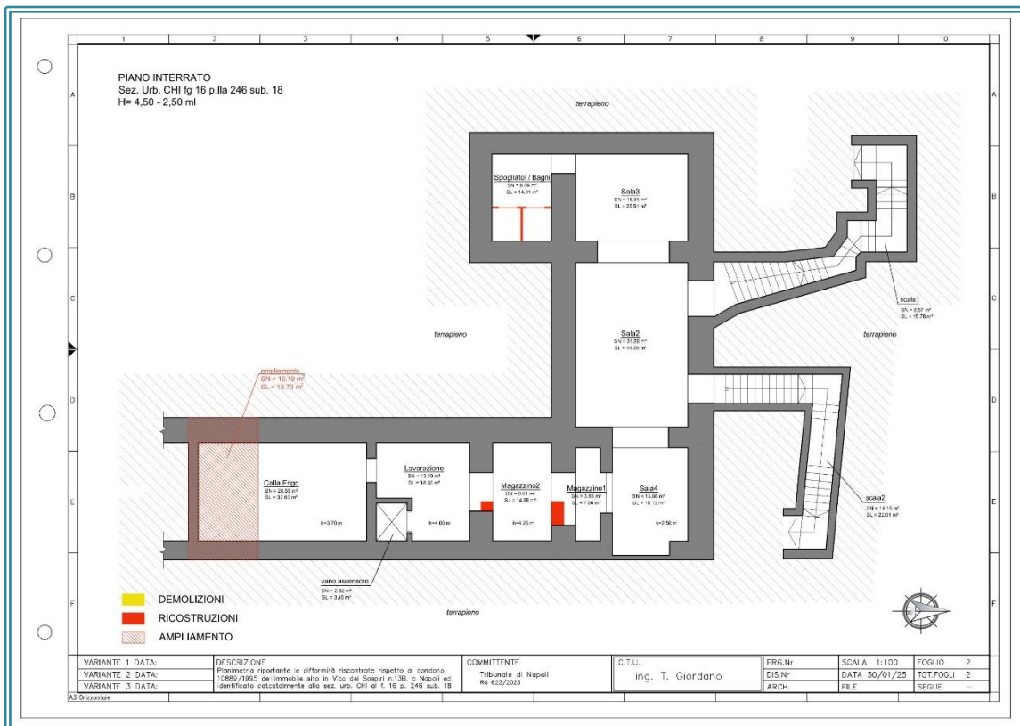
Figura 58 Schema difformità – Piano Interrato
