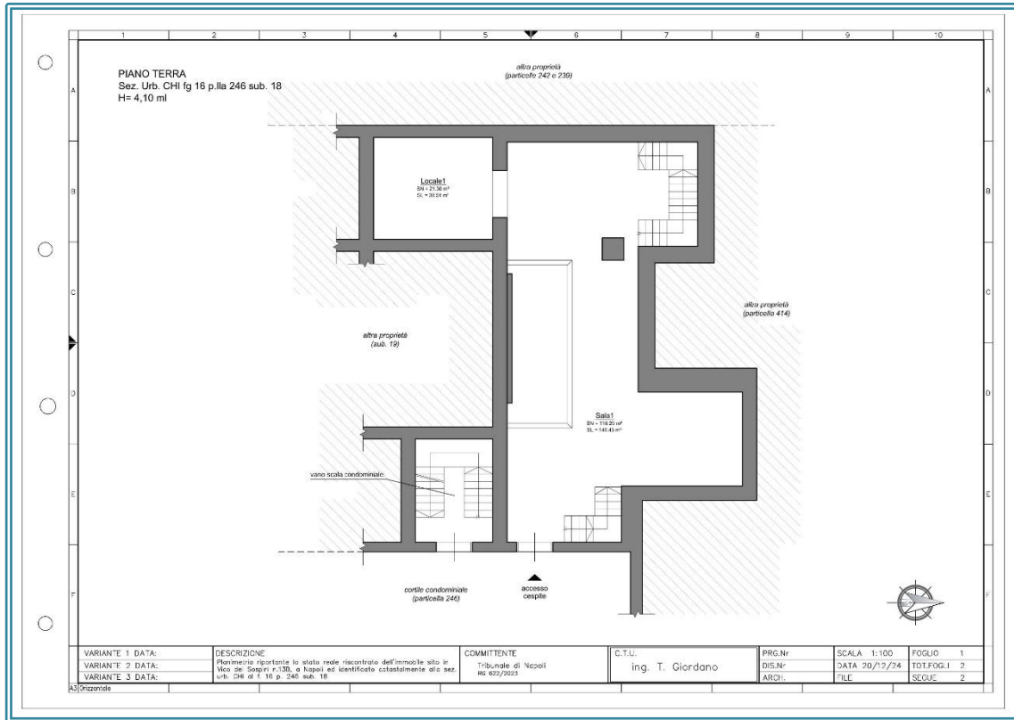
Figura 6 Piano Terra stato attuale
