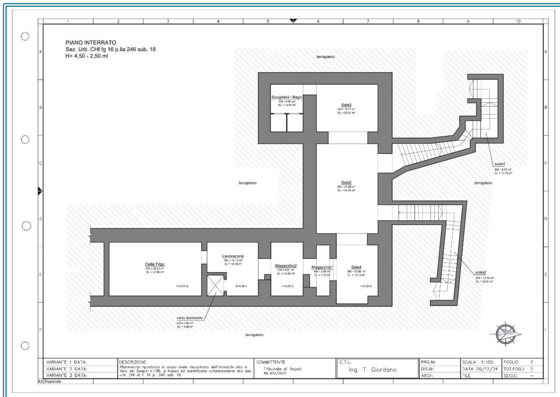
Figura 7 Piano interrato stato attuale
