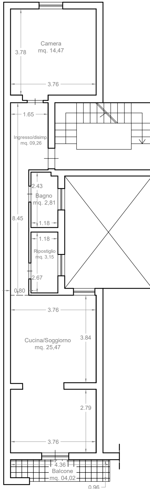
PIANTA APPARTAMENTO SC. 1:100
