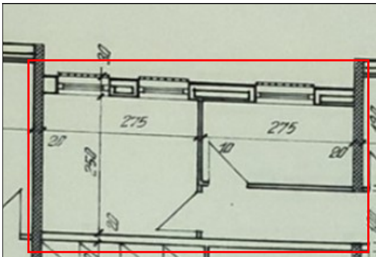
Planimetria delle cantine sub 21 e 22, allegata alla Concessione Edilizia di Variante in corso d'opera n. 44389/3750 del 22/5/1981
