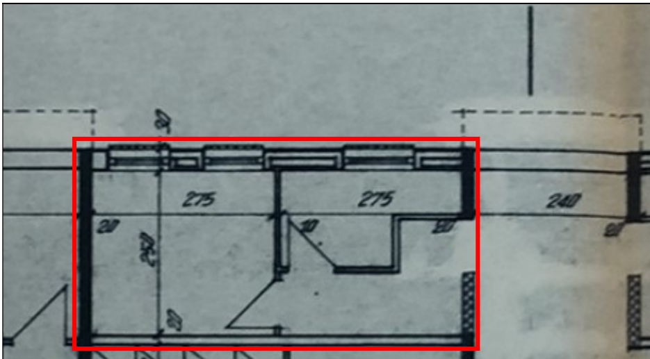
Planimetria delle cantine sub 21 e 22 nel grafico della Concessione Edilizia di Variante in corso d'opera n. 62723/6716 del 26/10/1985
