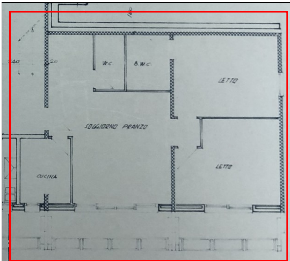
Planimetria dell'appartamento nel grafico della Concessione Edilizia di Variante in corso d'opera n. 62723/6716 del 26/10/1985
