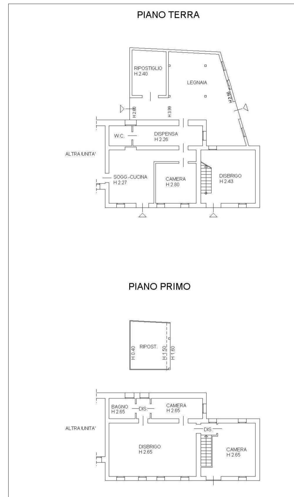
PLANIMETRIA CATASTALE sub. 2
