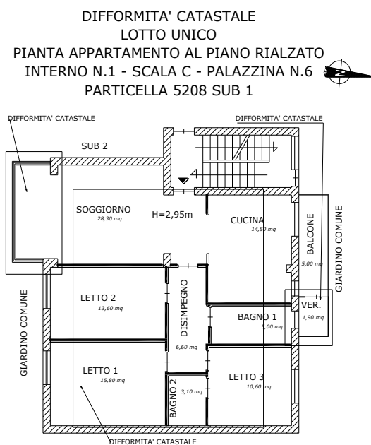
Figura 28 planimetria delle difformità catastali dell'appartamento al piano rialzato
