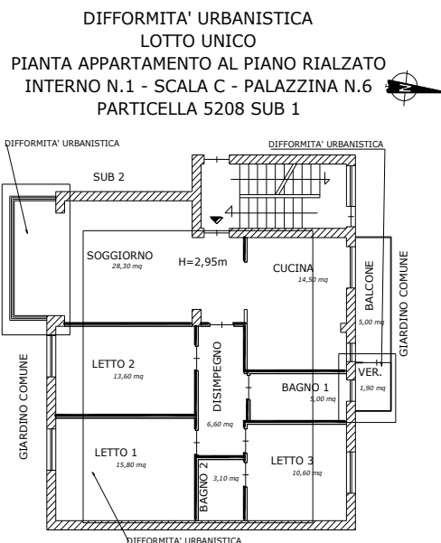
Figura 30 planimetria delle difformità urbanistiche dell'appartamento al piano rialzato
