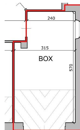
Planimetria box da SCIA n. 2021/79
