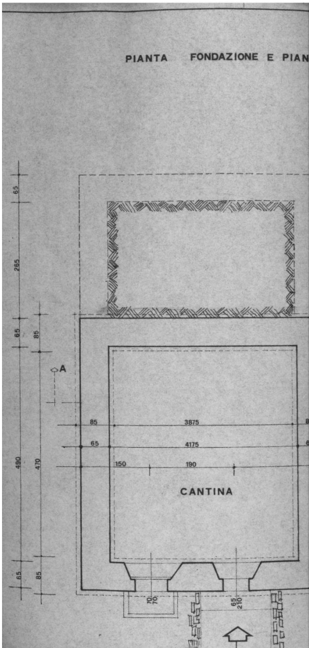
Figura 4 – Lotto 2 – misure del corpo CA
