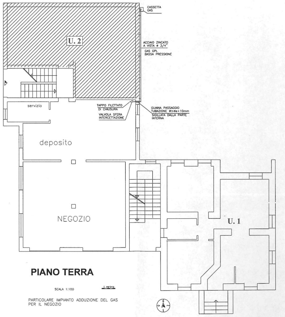
Figura 3 – Lotto 1 – misure del corpo A
