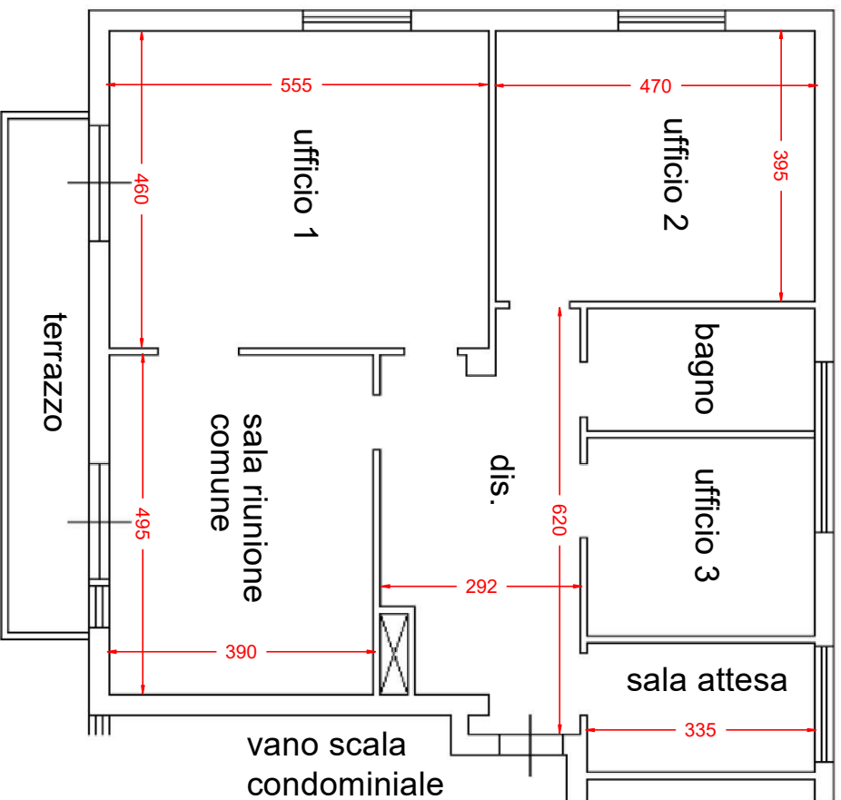
Piano 2° h=275 - Civitanova Marche F. 10 part. 927 sub 80
