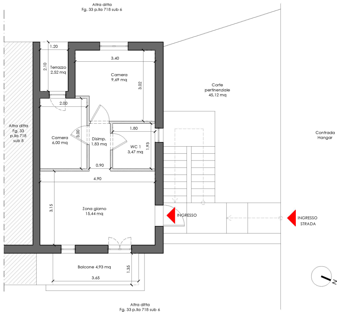
Figura 6: Rilievo Stato di fatto _ Pianta piano primo (Allegato 6D)
