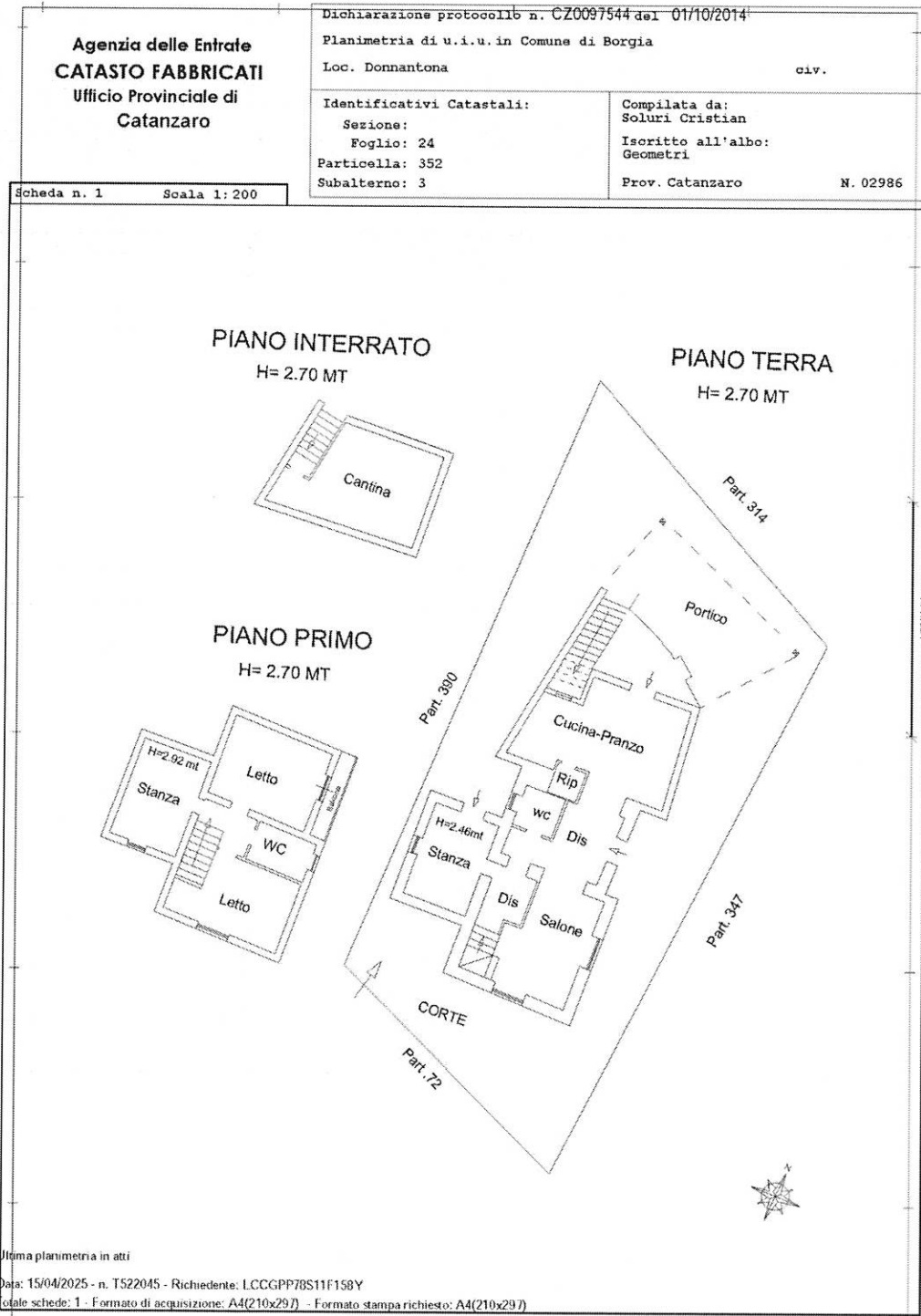
Immagine 5 - Planimetria catastale unità immobiliare censita al Foglio 24 Particella 352 Subalterno 3 del N.C.E.U. Comune di Borgia
