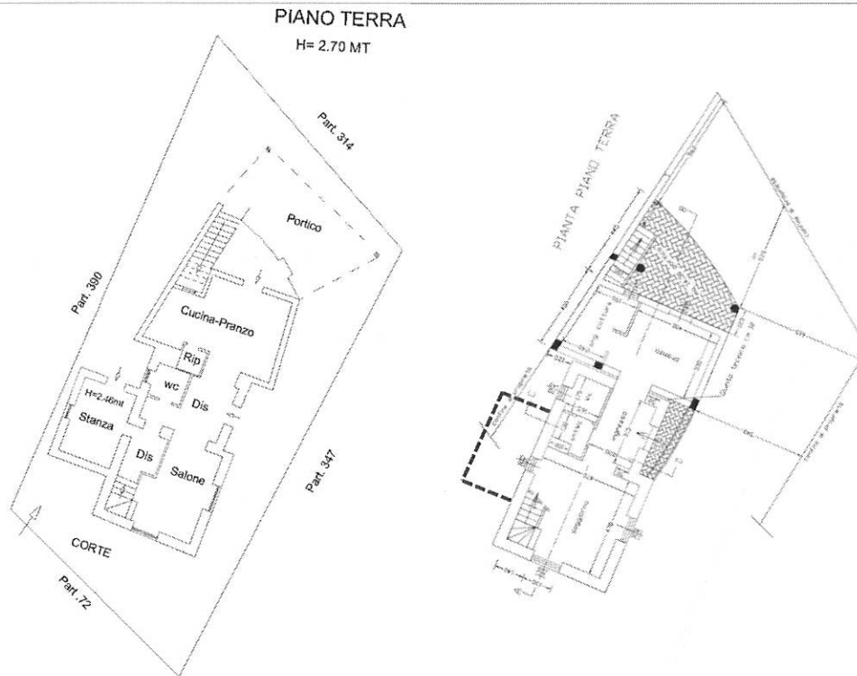
Immagine 8 - Piano Terra dell'unità immobiliare - Confronto tra planimetria catastale (a sinistra) e pianta di progetto allegata al Permesso di Costruire n. 2111 del 16/02/2004 (a destra)
