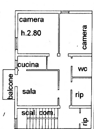
PIANO SECONDO
