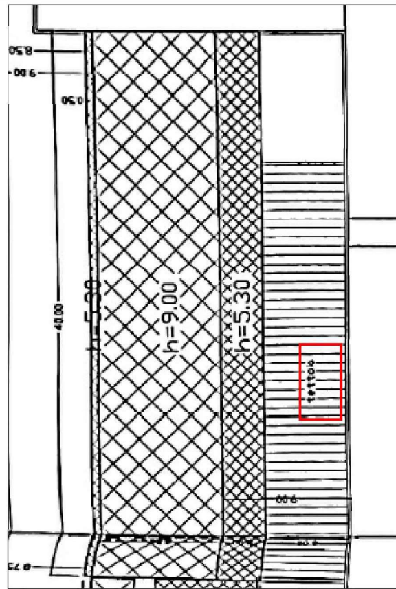
Stralcio planimetria di progetto allegata alla C.E. 21036/2000 - Fuori scala
