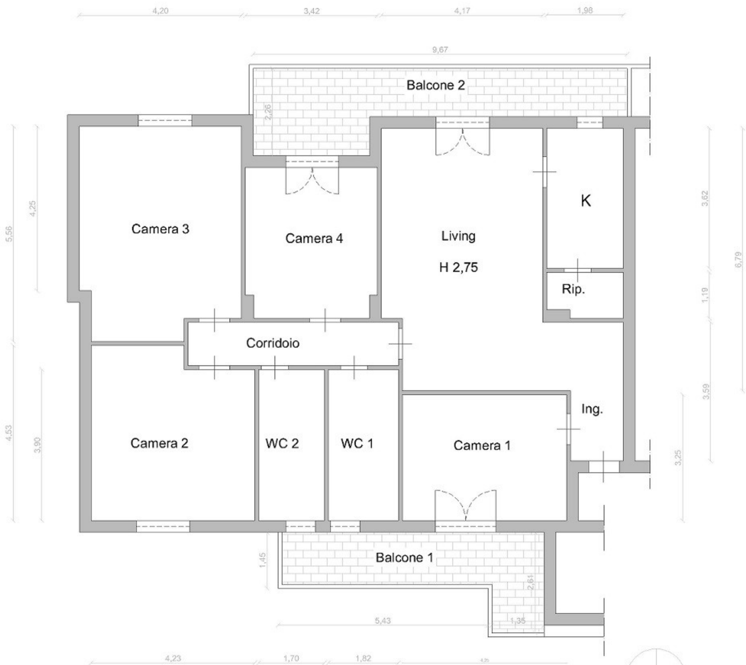
GRAFICI DI RILIEVO - APPARTAMENTO SITO AL SECONDO PIANO, SCALA B, INT. 7 - CASAPULLA (CE) VIA A. DIAZ. N. 48 - IN CATASTO AL FOGLIO 5, P.LLA 5001, SUB 37, CAT. A/2. - SCALA 1:100
