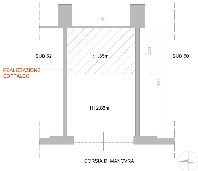
GRAFICI DI RILIEVO CON INDICAZIONE DELLE DIFFORMITA' CATASTALI - BOX AUTO SITO AL PIANO S1, SCALA B, - CASAPULLA (CE) VIA A. DIAZ, N. 48 - IN CATASTO AL FOGLIO 5, P.LLA 5001, SUB 51, CAT. C/6. - SCALA 1:100
