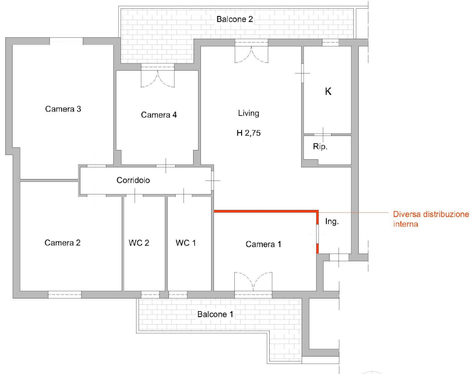
GRAFICI DI RILIEVO CON INDICAZIONE DELLE DIFFORMITA' CATASTALI - APPARTAMENTO SITO AL SECONDO PIANO, SCALA B, INT. 7 - CASAPULLA (CE) VIA A. DIAZ, N. 48 - IN CATASTO AL FOGLIO 5, P.LLA 5001, SUB 37, CAT. A/2. - SCALA 1:100
