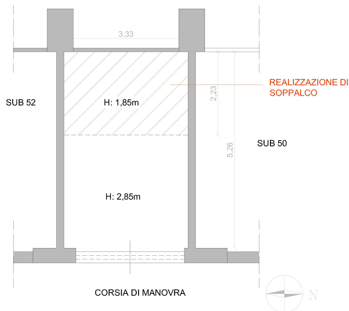
GRAFICI DI RILIEVO CON INDICAZIONE DELLE DIFFORMITA' EDILIZIE - BOX AUTO SITO AL PIANO S1, SCALA B, - CASAPULLA (CE) VIA A. DIAZ. N. 48 - IN CATASTO AL FOGLIO 5, P.LLA 5001, SUB 51, CAT. C/6. - SCALA 1:100
