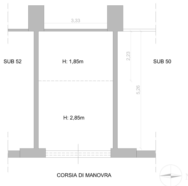
GRAFICI DI RILIEVO - BOX AUTO SITO AL PIANO S1, SCALA B, - CASAPULLA (CE) VIA A. DIAZ, N. 48 - IN CATASTO AL FOGLIO 5, P.LLA 5001, SUB 51, CAT. C/6. - SCALA 1:100
