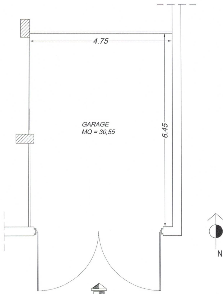
Figura 6 - Planimetria Catastale Foglio 23, p.lla 371, sub 5 (ex sub 2) – Piano S1
