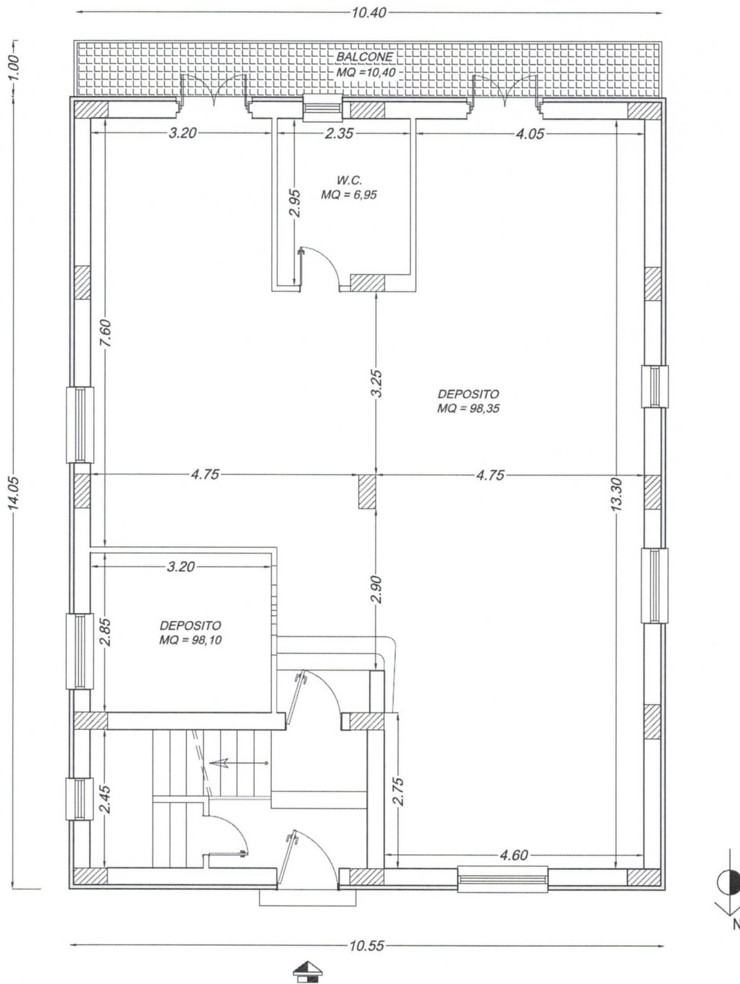
Figura 9 - Planimetria Catastale Foglio 23, p.lla 371, sub 7 (ex sub 3) - Piano T
