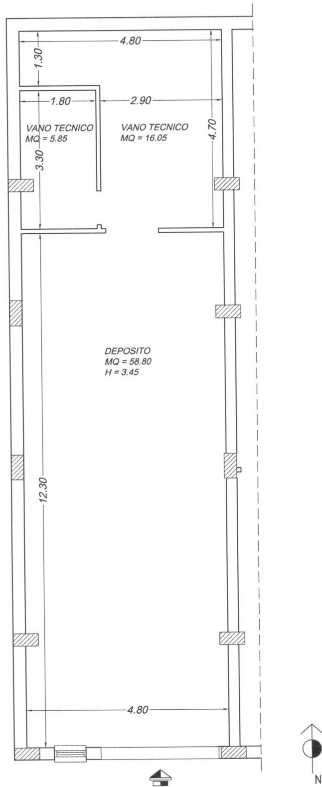
Figura 10 - Planimetria Stato di fatto Foglio 23, p.lla 371, sub 6 (ex sub 2) – Piano S1
