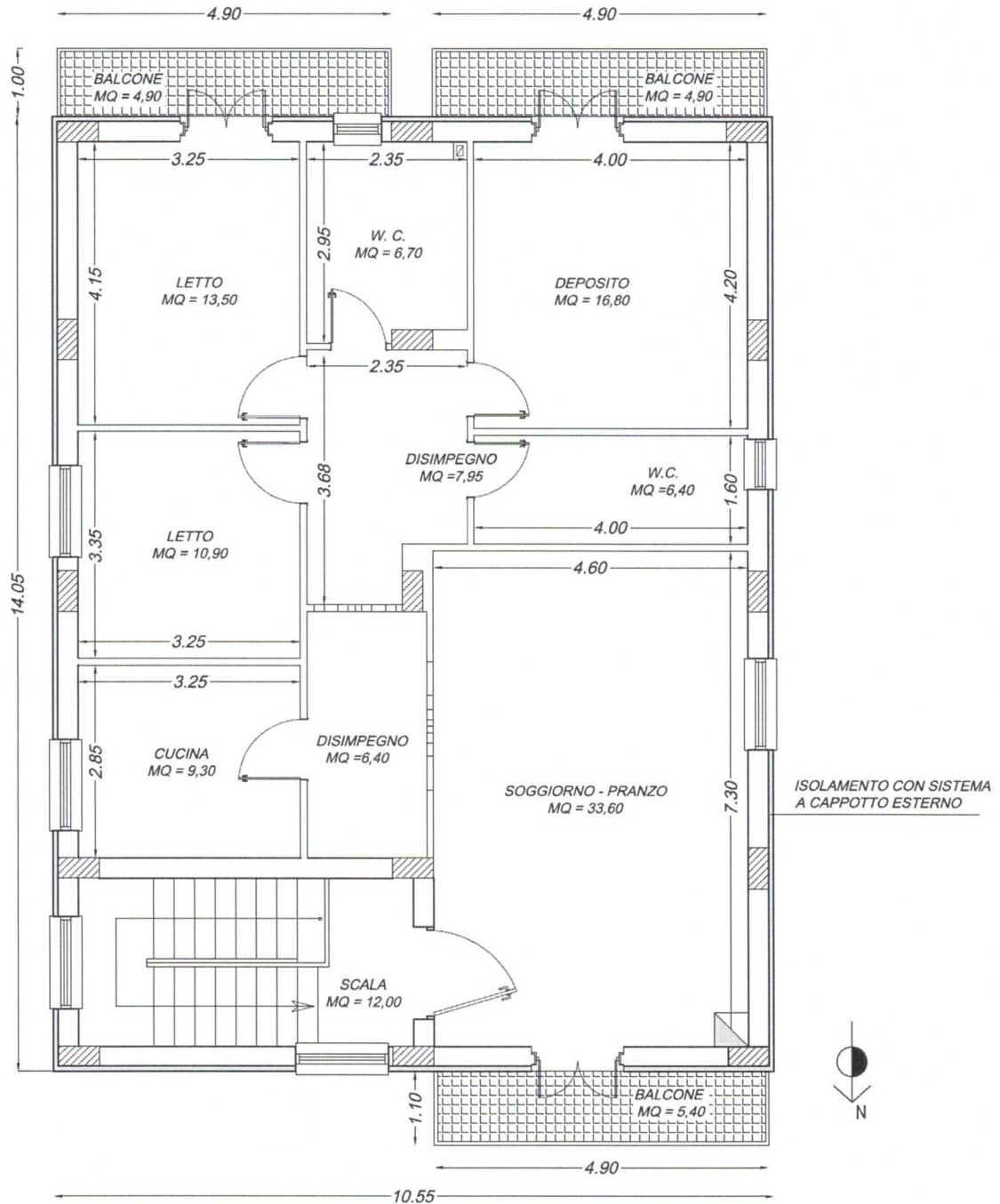
Figura 5 - Planimetria Catastale Foglio 23, p.lla 371, sub 4 – Piano Primo
