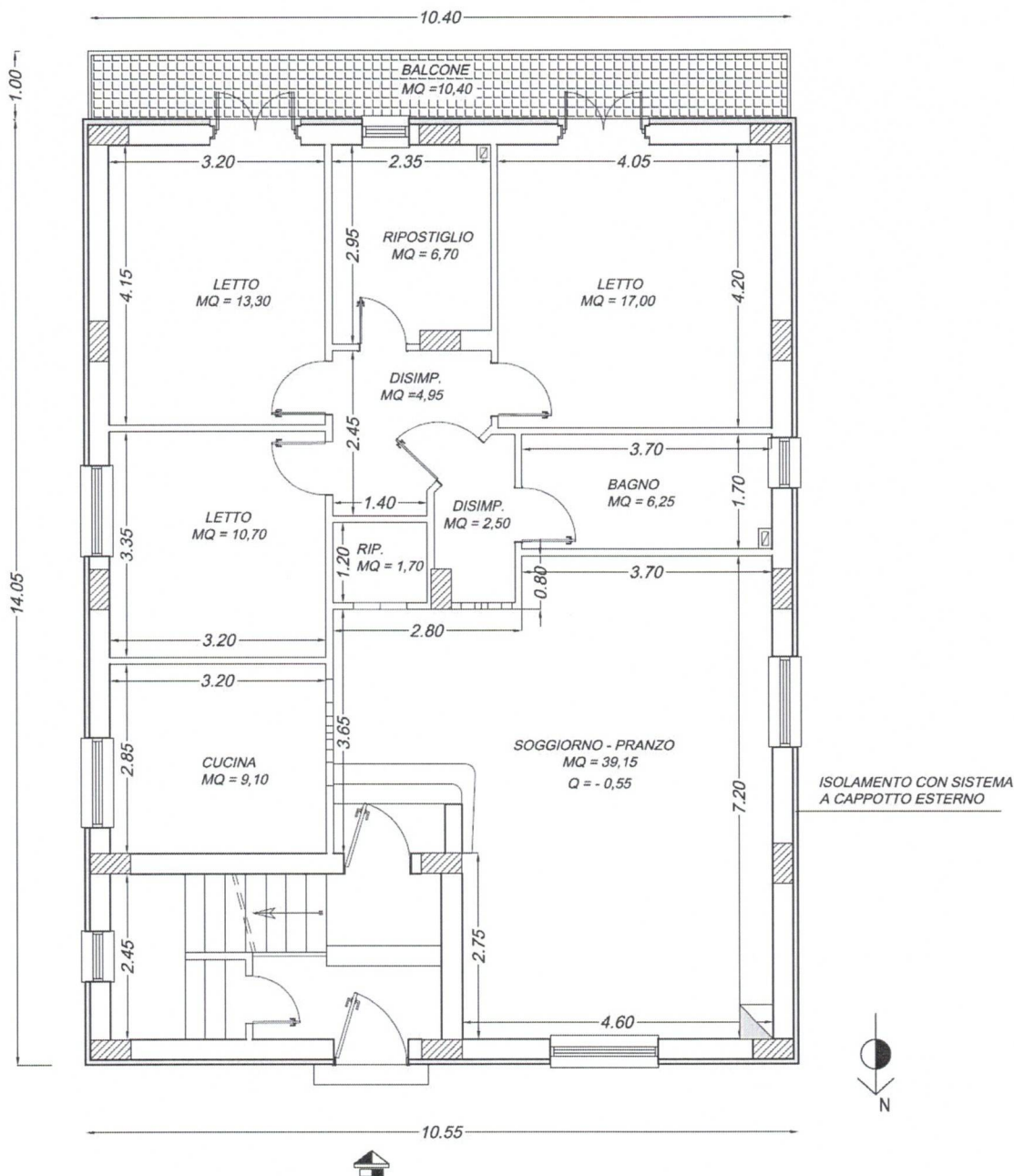
Figura 11 - Planimetria Stato di fatto Foglio 23, p.lla 371, sub 7 (ex sub 3)
