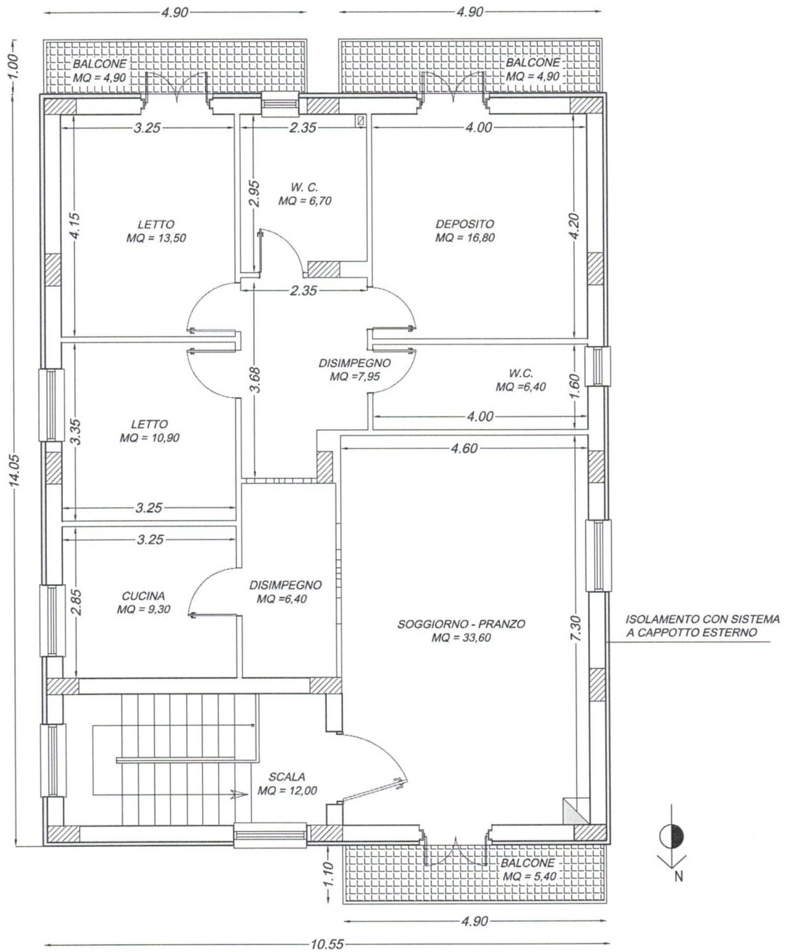
Figura 7 - Planimetria Stato di Fatto Foglio 23, p.lla 371, sub 4 - Piano Primo
