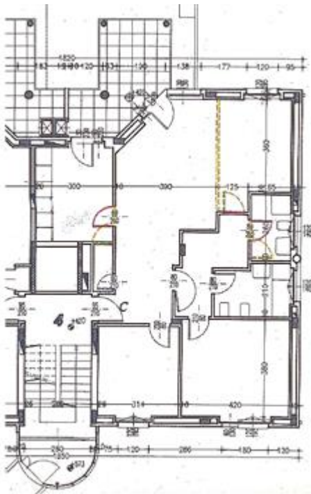
planimetria dell'alloggio a piano 1° - stato autorizzato
