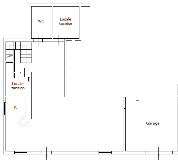
Planimetria di piano seminterrato
