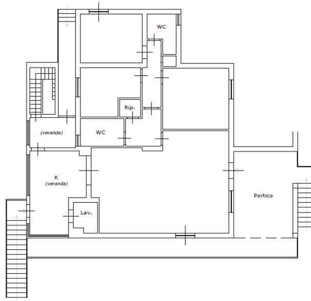
Planimetria di piano terra
