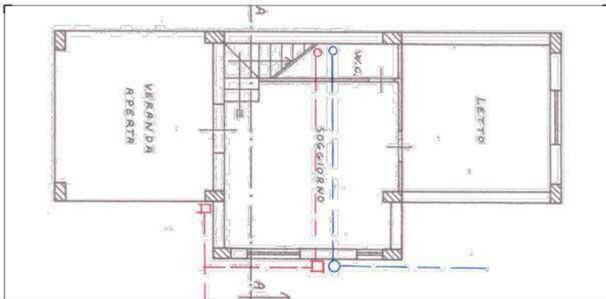
Situazione assentita al Comune – Piano Terra
