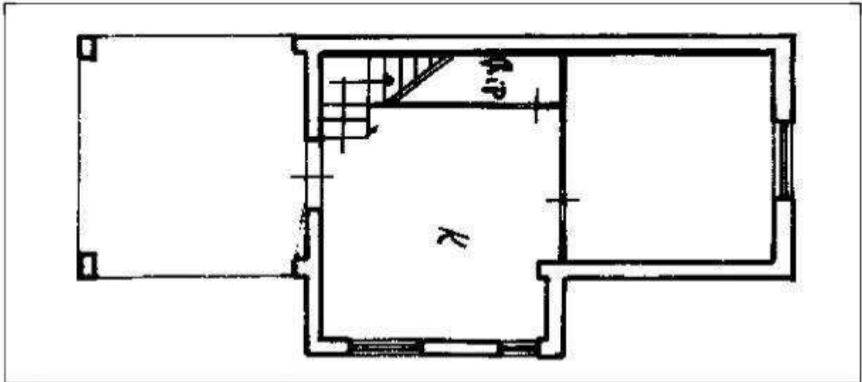
Planimetria Catastale – Piano Terra
