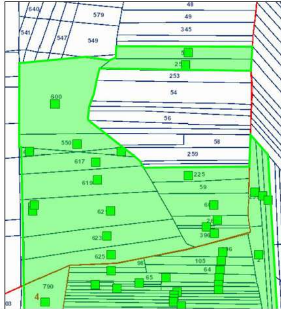
STRALCIO DI MAPPA CATASTALE
