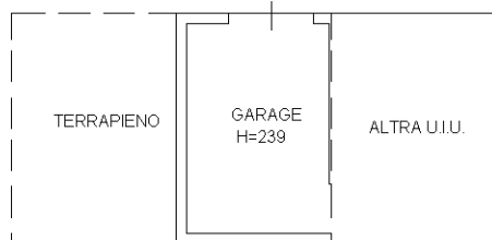
PIANTA PIANO SEMINTERRATO
