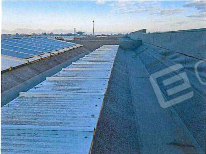
Foto 145 - Copertura lato S-O .jpg
