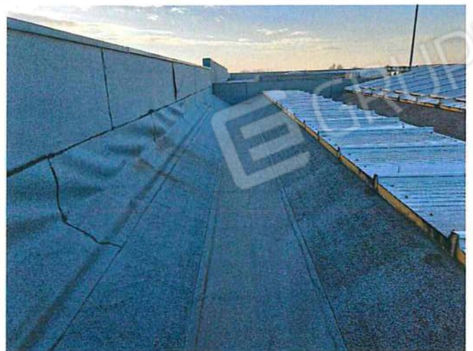
Foto 162 - Copertura lato S-E.jpg
