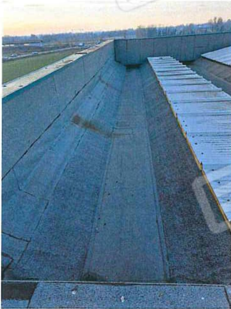
Foto 139 - Copertura lato S-O.jpg
