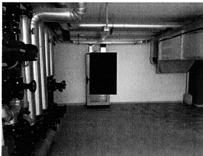
Foto n. 50 – Piano soppalco - locale unità trattamento aria
