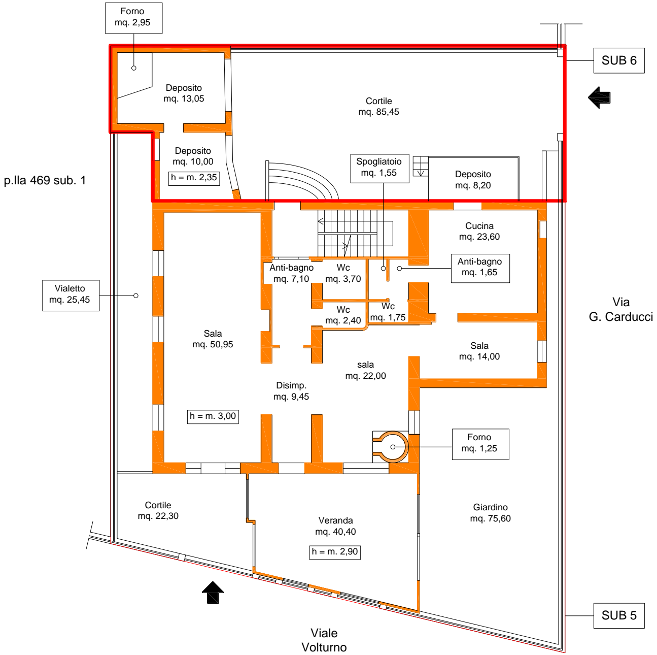
Rilievo del piano terra
