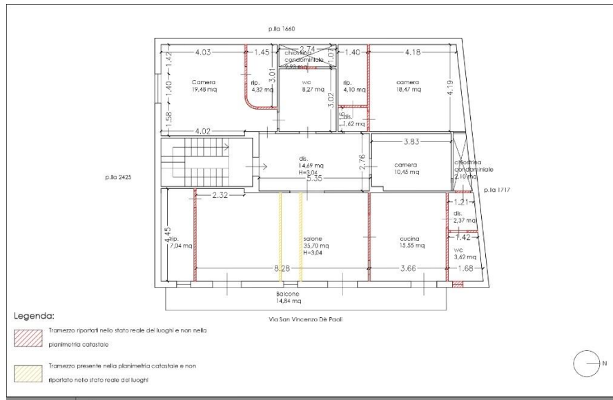
ALL. 7 PLANIMETRIA STATO REALE DEI LUOGHI CON INDICAZIONE GRAFICA DELLE DIFFORMITÀ RISCOSETRATE RISPETTO ALLA PLANIMETRIA CATASTALE ARCH. CAROLINA TARAGNOLINI scala 1:100
