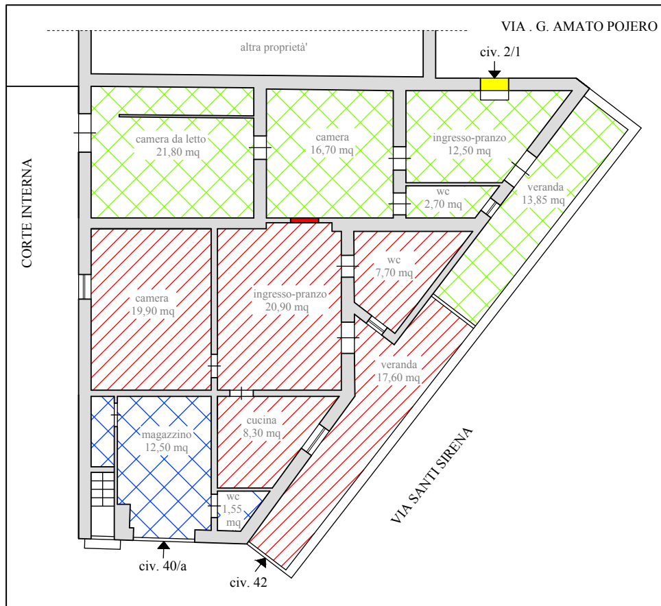
Planimetria di rilievo dello stato di fatto con indicazione della divisione delle unità immobiliari
