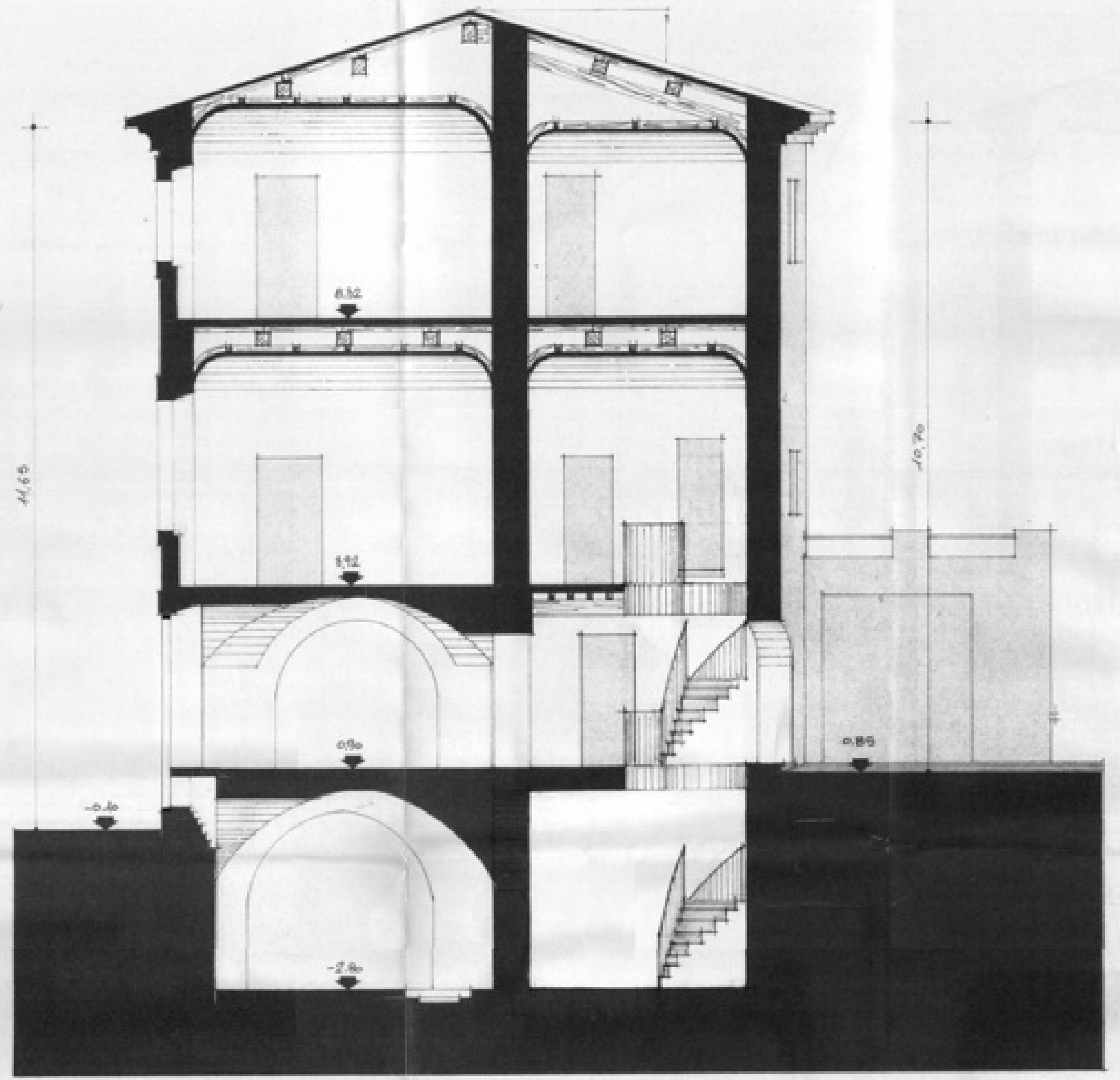
SEZIONE C-C
