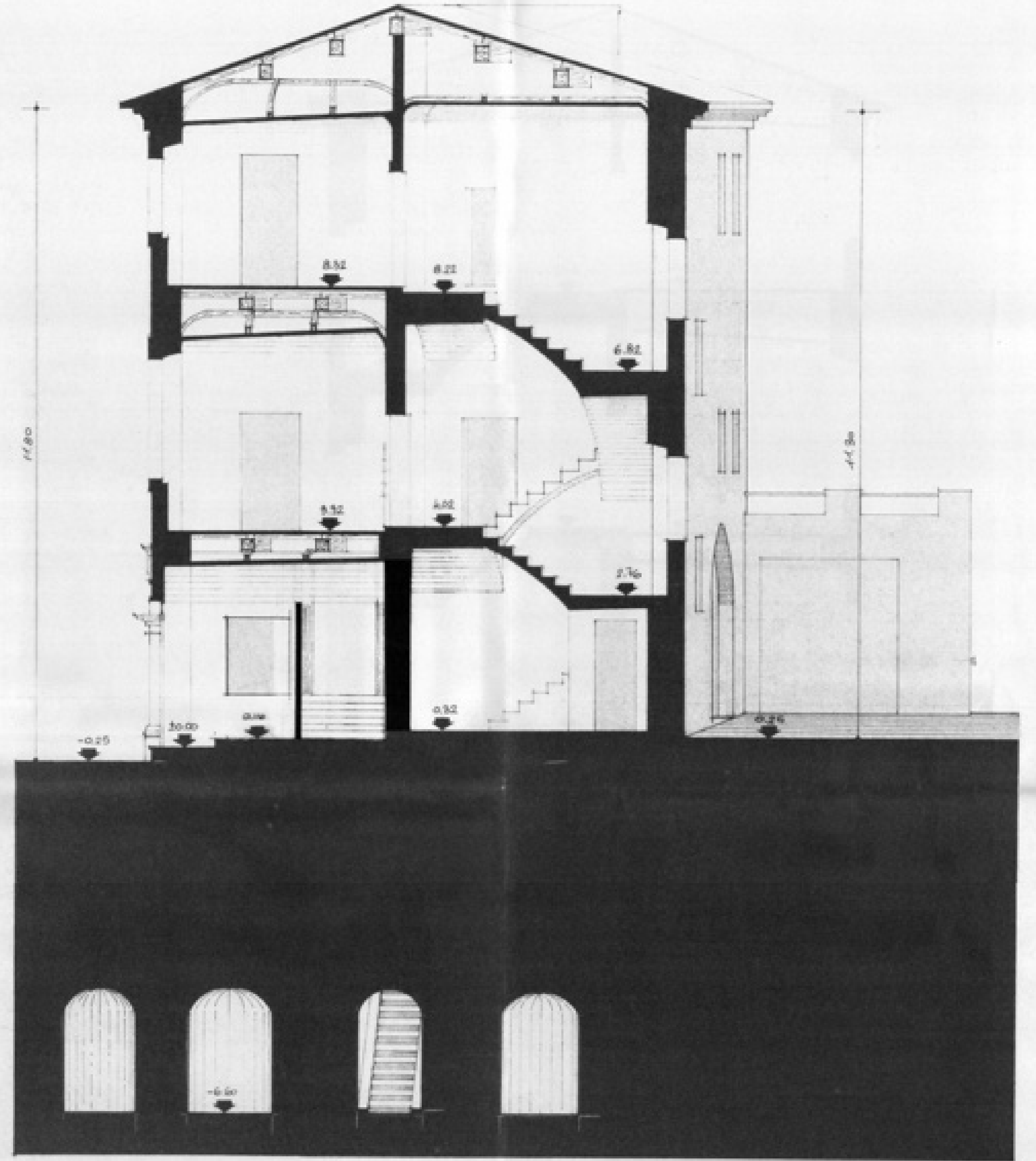
SEZIONE A-A
