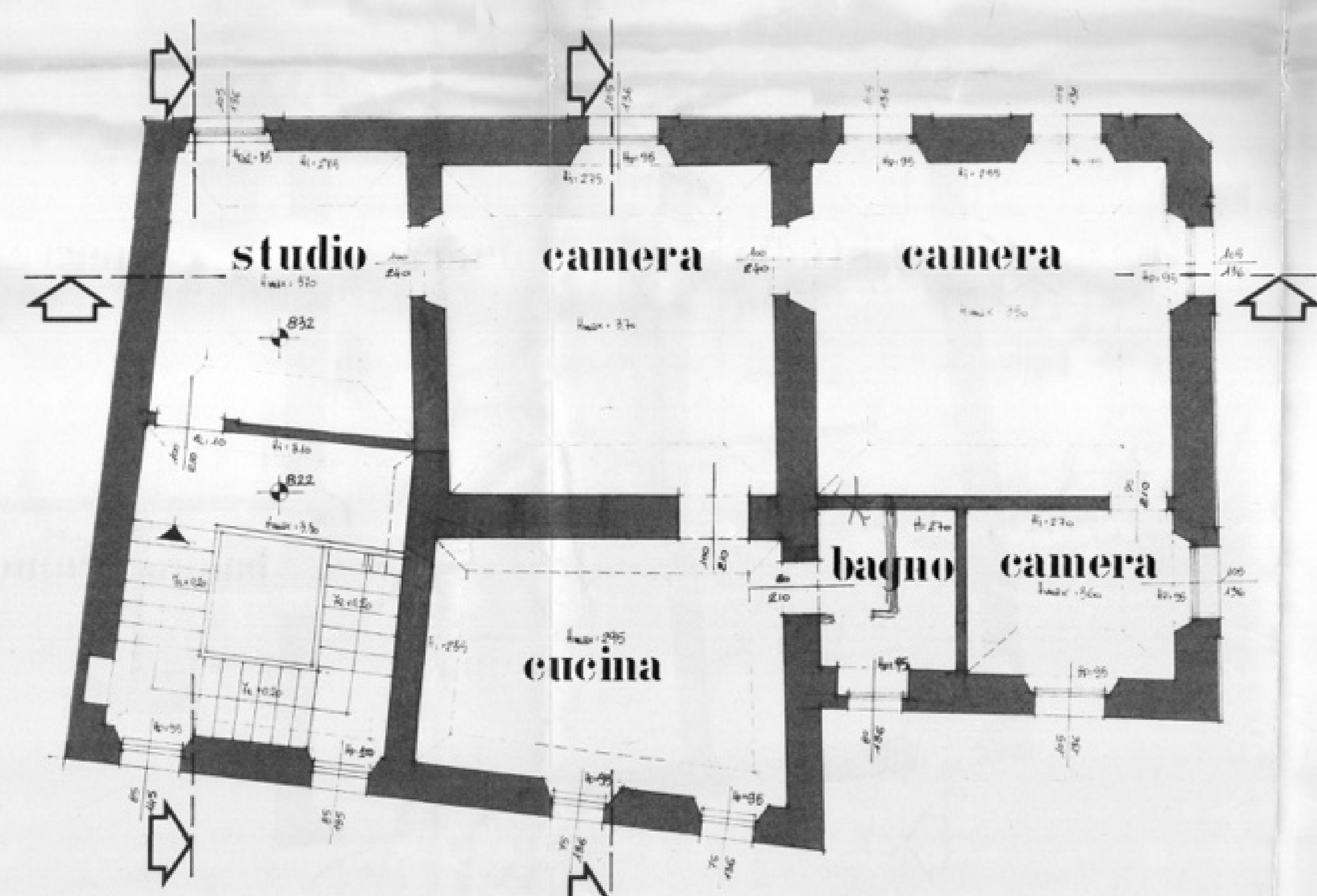
PIANO TERZO
