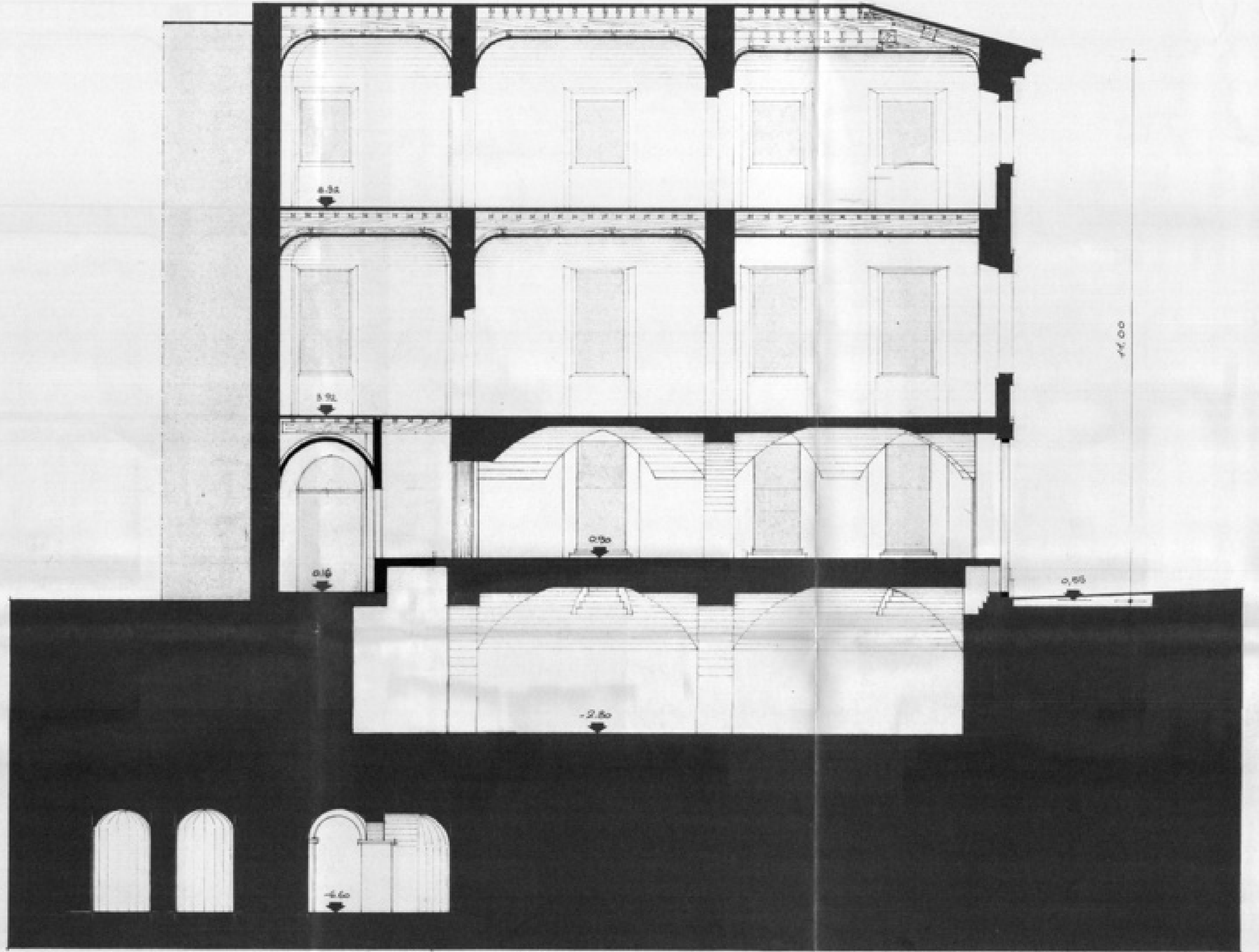
SEZIONE B-B
